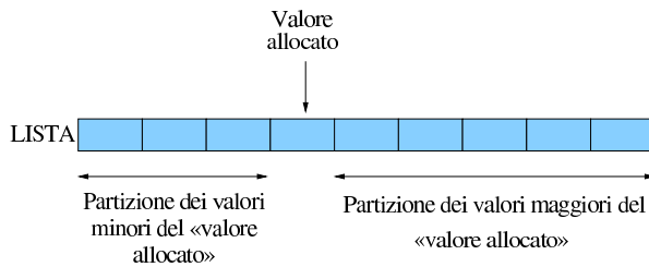
Figura 62.33. Il concetto base dell'algoritmo del Quicksort: suddivisione dell'array in due gruppi disordinati, separati da un valore piazzato correttamente nel suo posto rispetto all'ordinamento.
