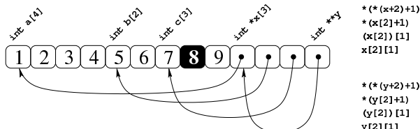
Figura 66.218. Tanti modi alternativi per raggiungere lo stesso elemento.
