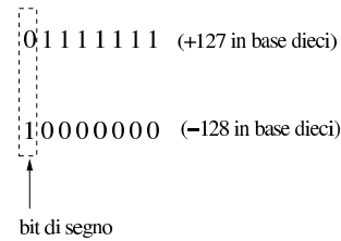
Figura 63.25. Valori massimi rappresentabili con soli otto bit.
