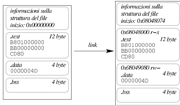
Figura 65.29. Dalle sezioni del file oggetto rilocabile ai segmenti del file oggetto eseguibile.
