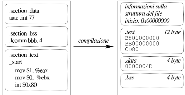
Figura 65.26. Dalle sezioni del file sorgente a quelle del file oggetto rilocabile.
